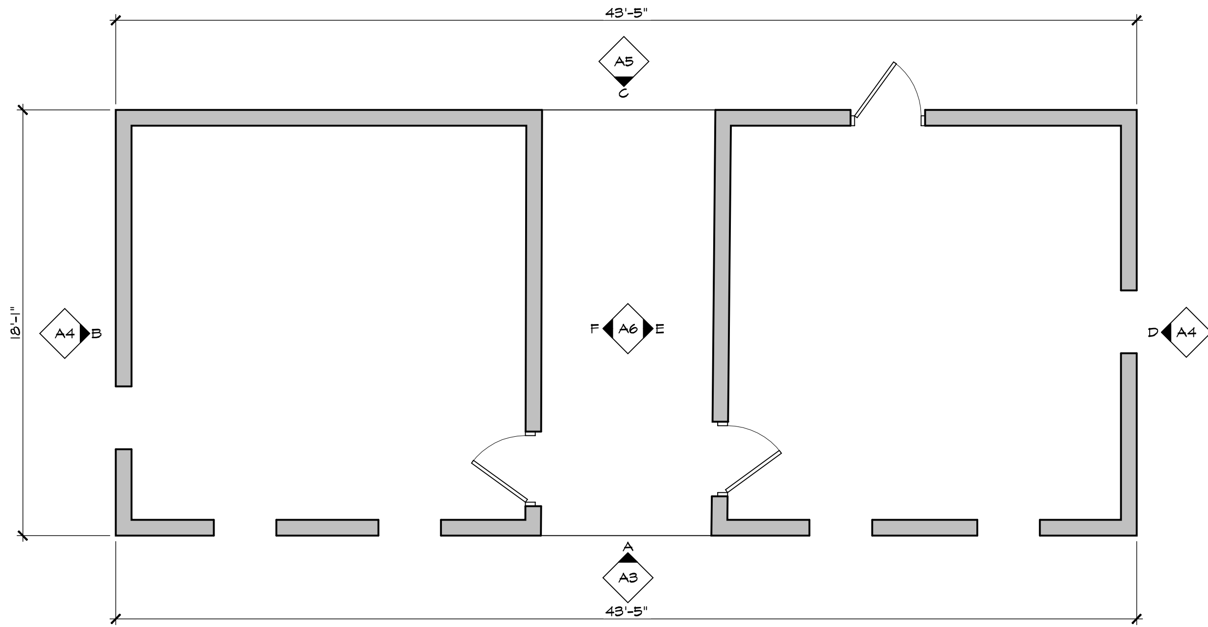
FIRST FLOOR PLAN N.T.S.
