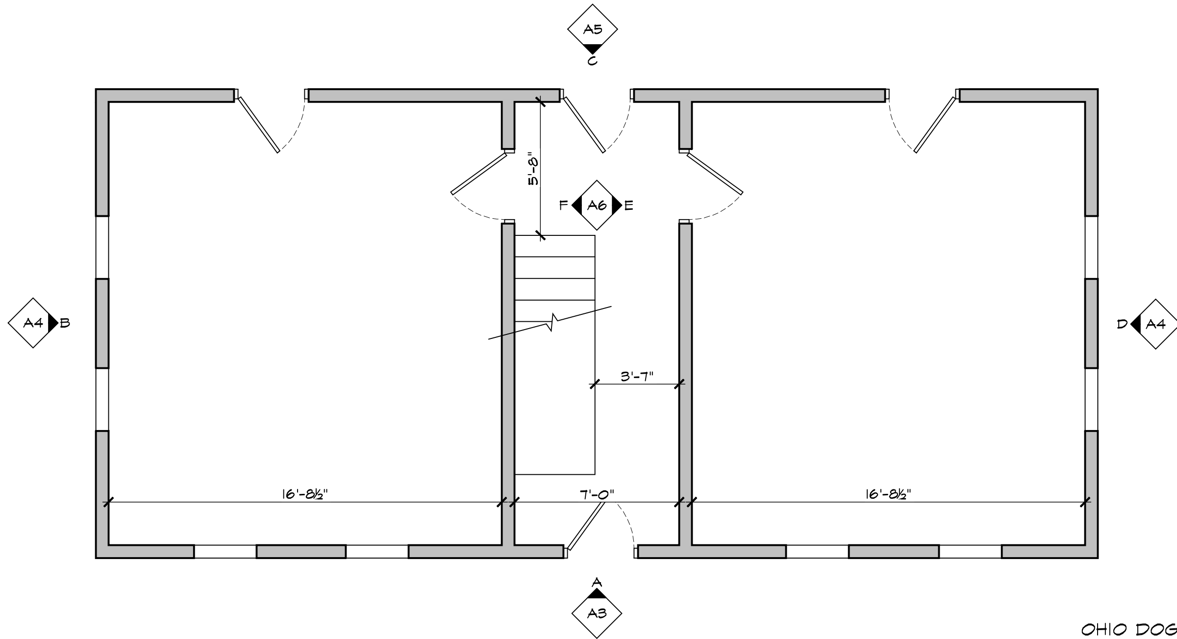
FIRST FLOOR PLAN N.T.S.
